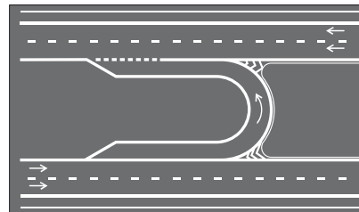
Ordenação de movimentos em retornos com faixa adicional para o movimento
