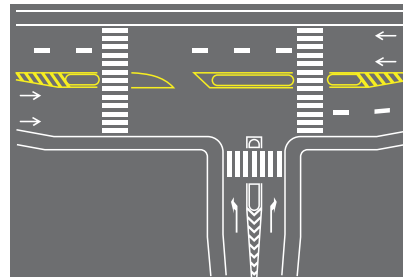
Ordenação de movimentos em retornos com faixa adicional para o movimento
