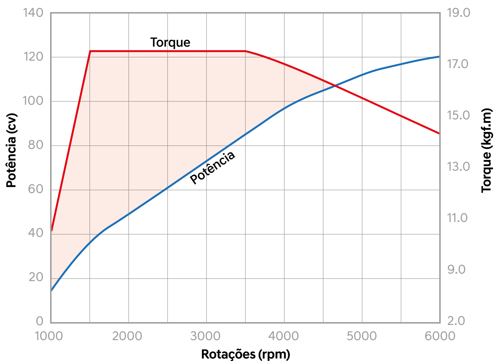
Relação potência x torque - motor Kappa 1.0 TGD (com etanol)
